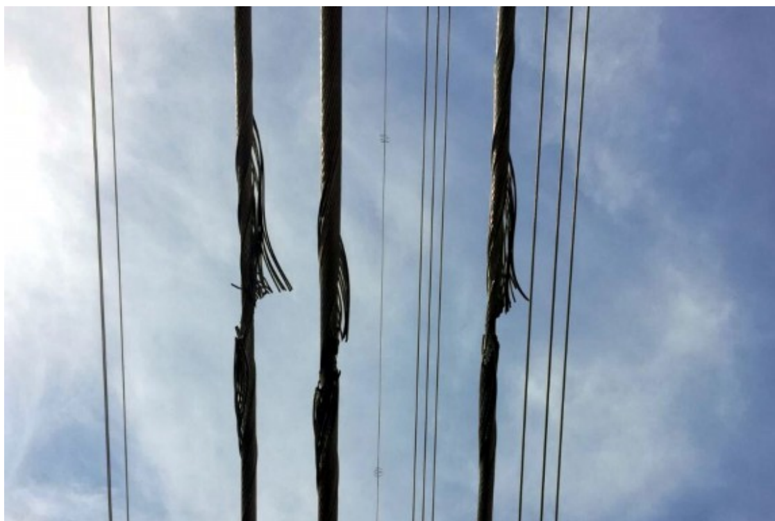
Els tres cables de la MAT a l'alçada de Cervià de Ter, desfilats després de rebre els impactes Foto: ACN.
